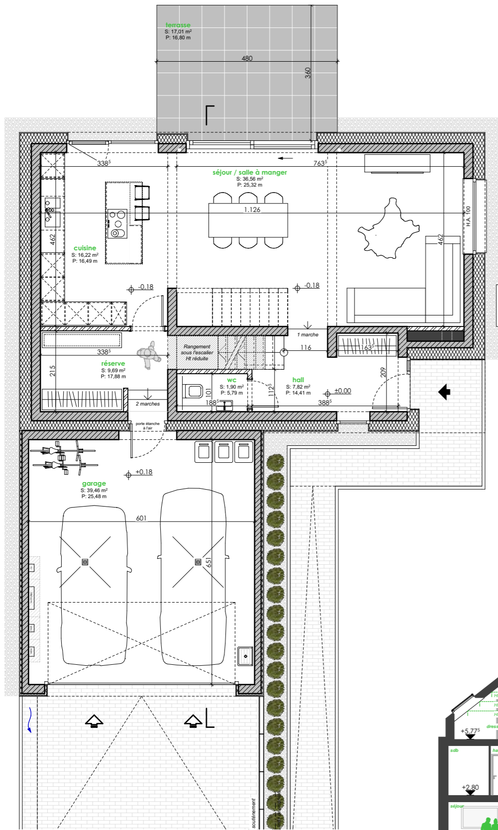
Rez-de-chaussée
