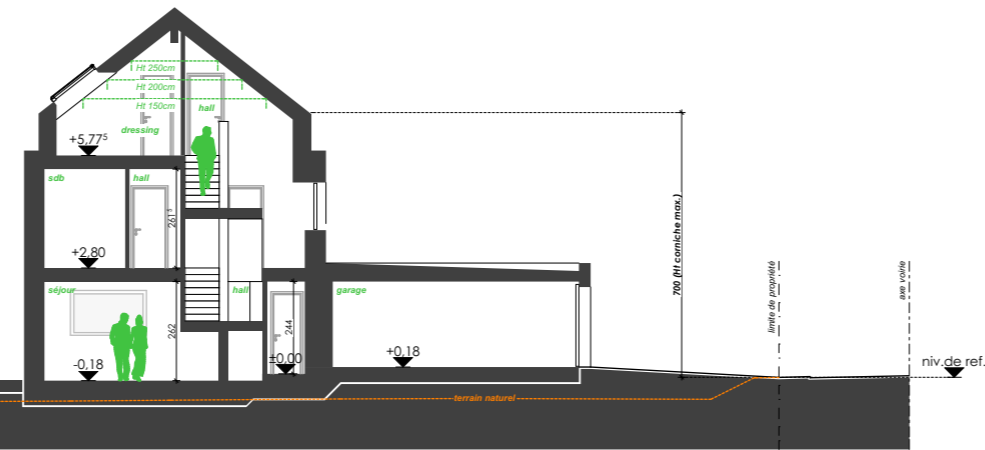
Coupe de principe (éch. 1/200)
