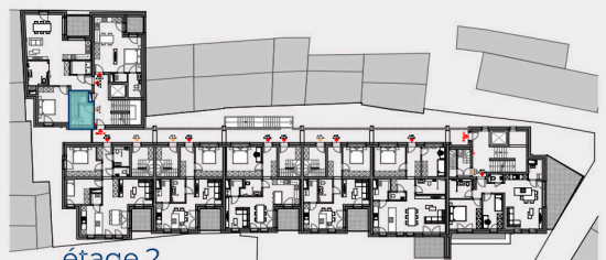
étage 2
